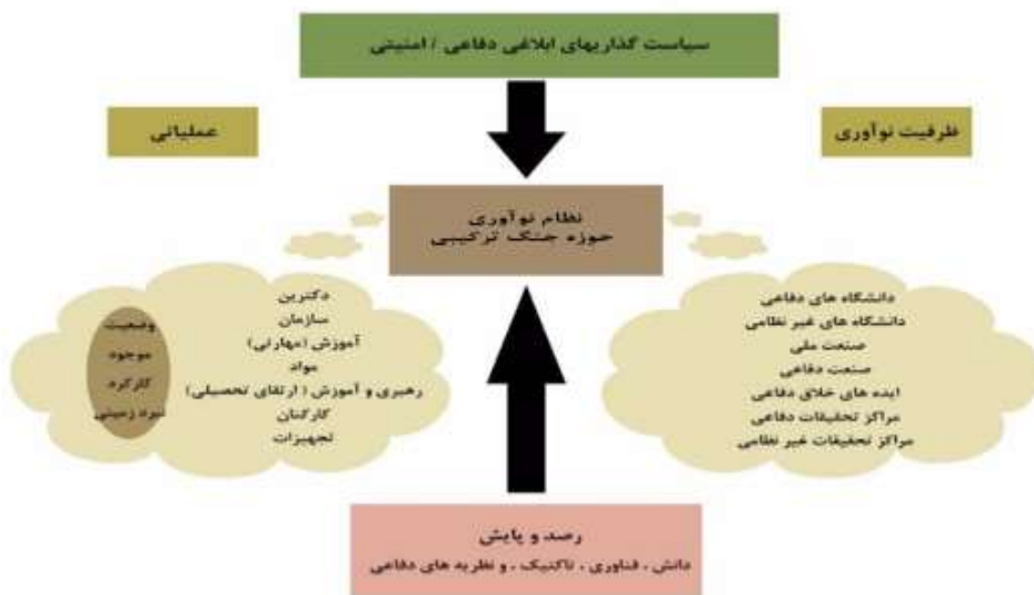
شکل ۶: مدل مفهومی
