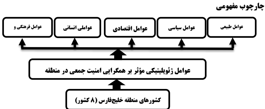
شکل ۳: چارچوب نظری
