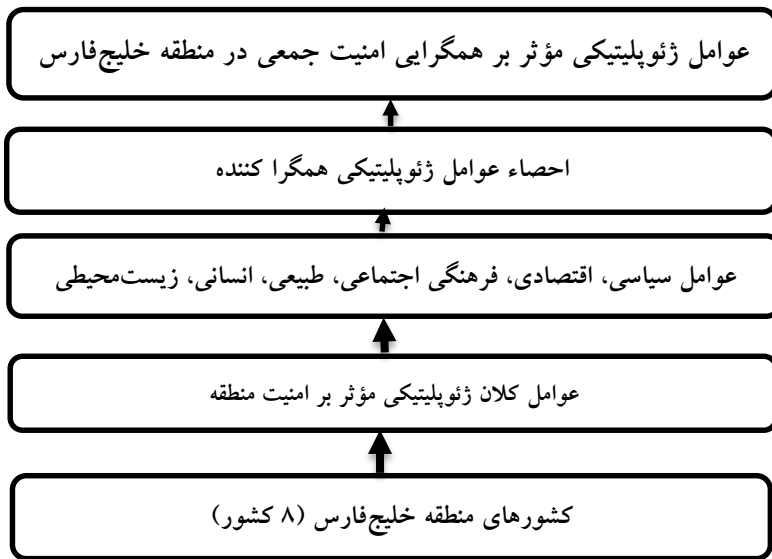
شکل ۳: چارچوب نظری
